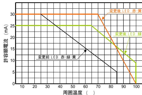
許容順電流-周囲温度
