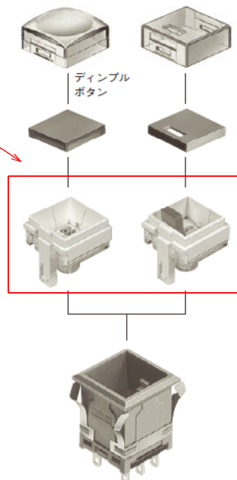
参考図 (EH形)
